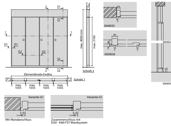
EI30 RF1 VKF NR. 23094
