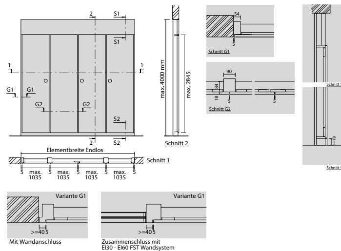
EI30 RF1 VKF NR. 23098
