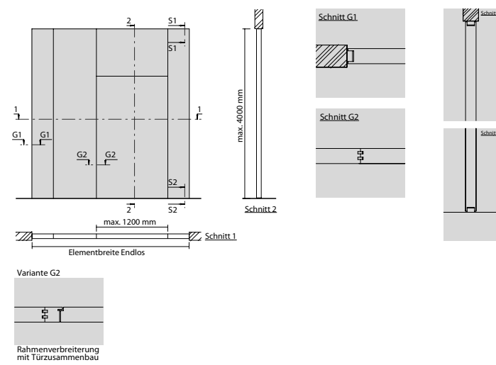
EI90 RF1 VKF NR. 24544
