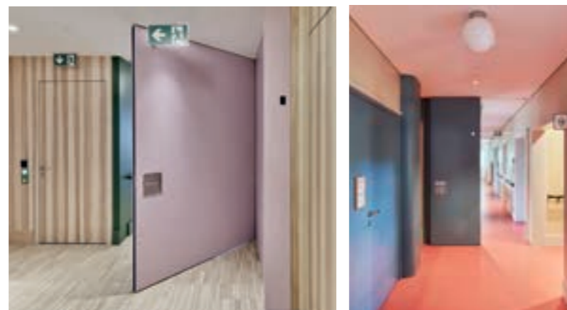
Porte coupe-feu à pivot sans (à gauche) et avec vantail rabattable (à droite)
