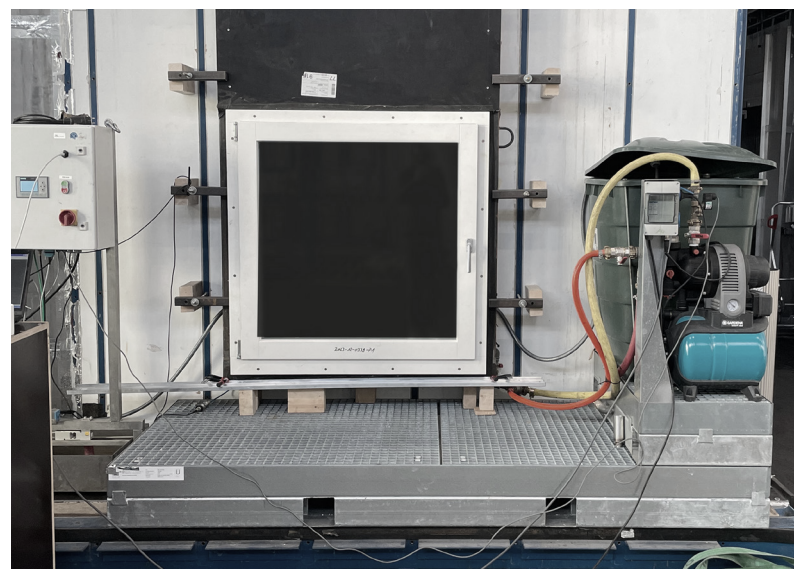
Lichtschachtfenster in Vorrichtung wird mit 1800 mm Wasserhöhe überflutet
