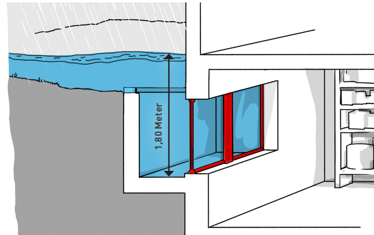
Skizze zeigt Lichtschachtfenster während eines Hochwassers
