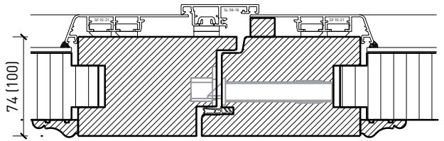
Mittelanschlag 74 / 100 mm, Türe gefälzt
