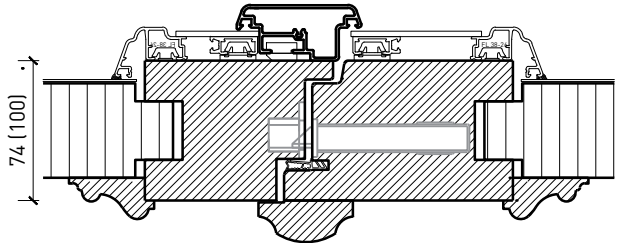
Mittelanschlag 74 / 100 mm, Schlagleisten profiliert
