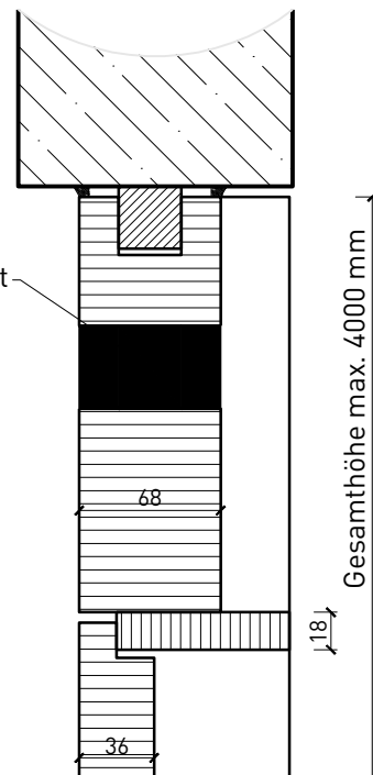
Deckenanschluss Schachtfrost in FeuerschutzTeam Vollwand
