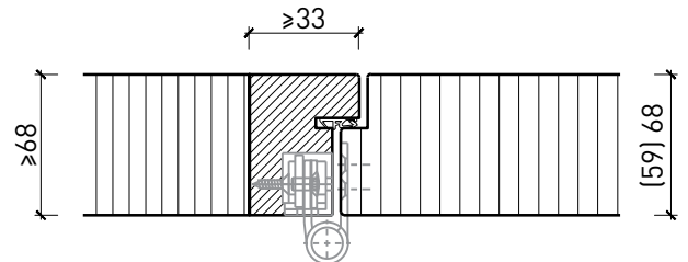
Einbau in Vollwand, Türe stumpf
