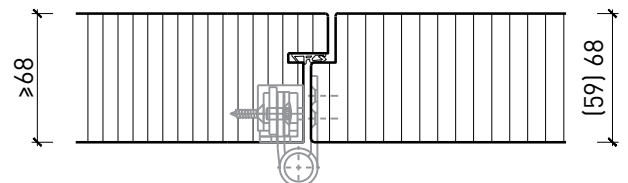
Einbau in Vollwand, Türe stumpf
