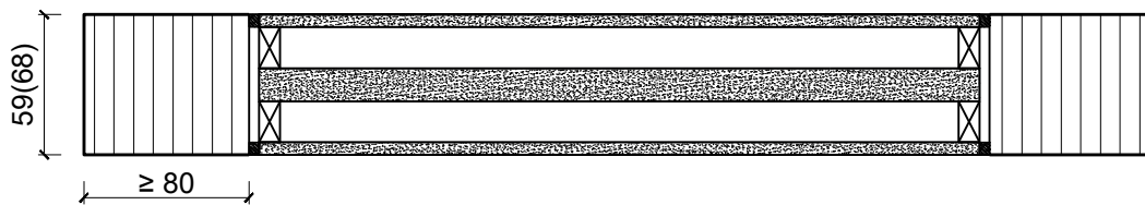
Plano-Verglasung
