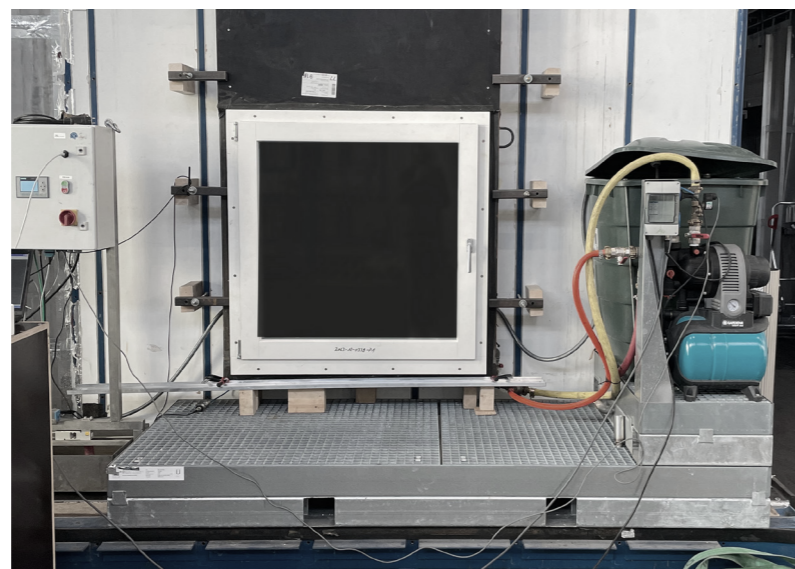
La fenêtre pour soupirail dans le dispositif est inondée avec une hauteur d'eau de 1 800 mm
