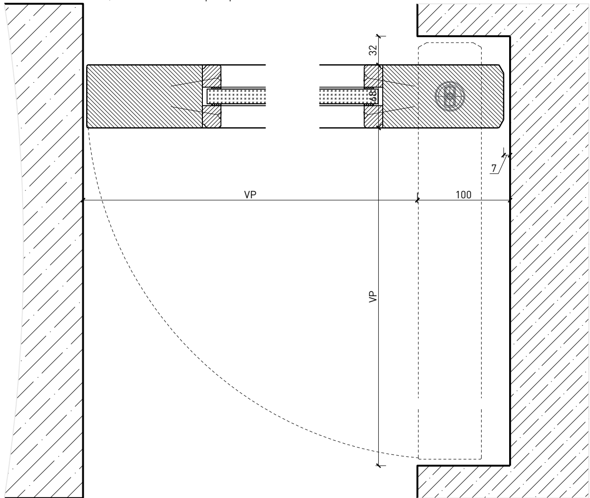
Porte battante sans cadre, avec renforcement pour position ouverte affleurant au mur
