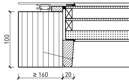
Profil en aluminium lisse parclose biseauté avec feuillure décoratif
