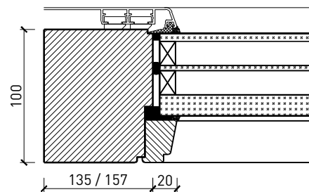
Profil en aluminium lisse parclose biseauté avec feuilure décoratif
