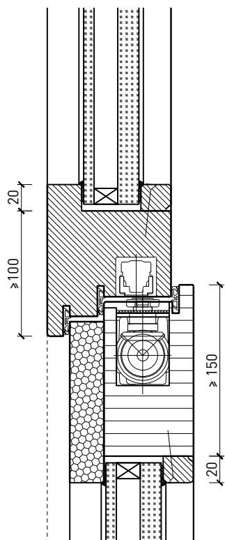
Porte avec doublage acoustique / imposte vitrée* Ferme-porte intégré*
