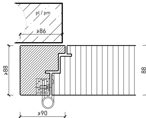
Cadre applique 88 mm, porte affleurée
