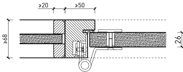
Intégration dans un vitrage fixe avec parcloles vissées
