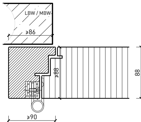
Blendrahmen 88 mm, Türe stumpf
